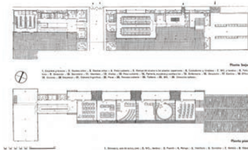
Figura 3: Planta baja y tipo del grupo escolar en la Av. Bogatell. Sert
