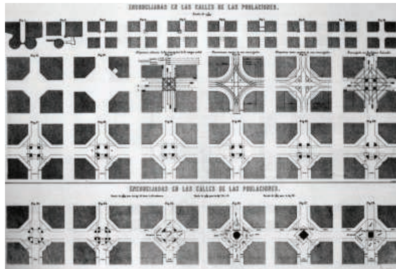
Figura 1: Estudio hecho por Cerdá para solucionar los refugios peatonales en los cruces
