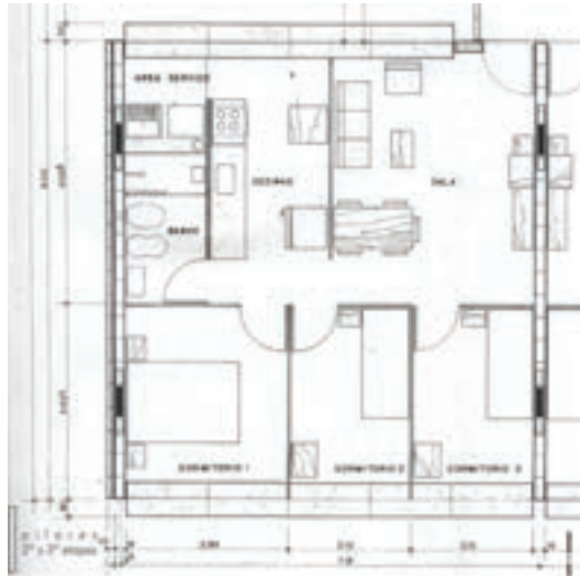
Figura 16. Planta de la unidad de vivienda
