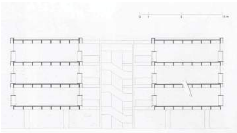
Figura 21. Sección bloque 1ª etapa
