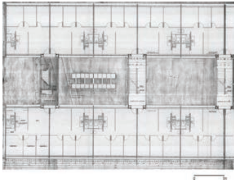
Figura 13. Planta del piso tipo 3ª etapa
