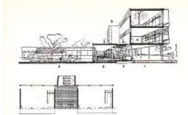
Figura 5: Sección transversal y aulas tipo. Proyecto de la escuela Kappeli. Roth
