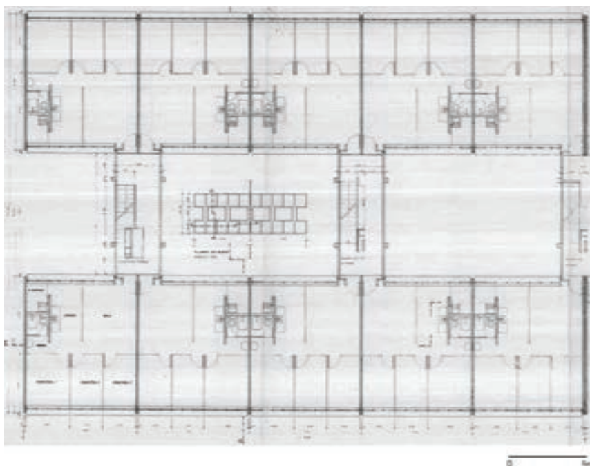
Figura 10. Planta del piso tipo 2ª etapa
