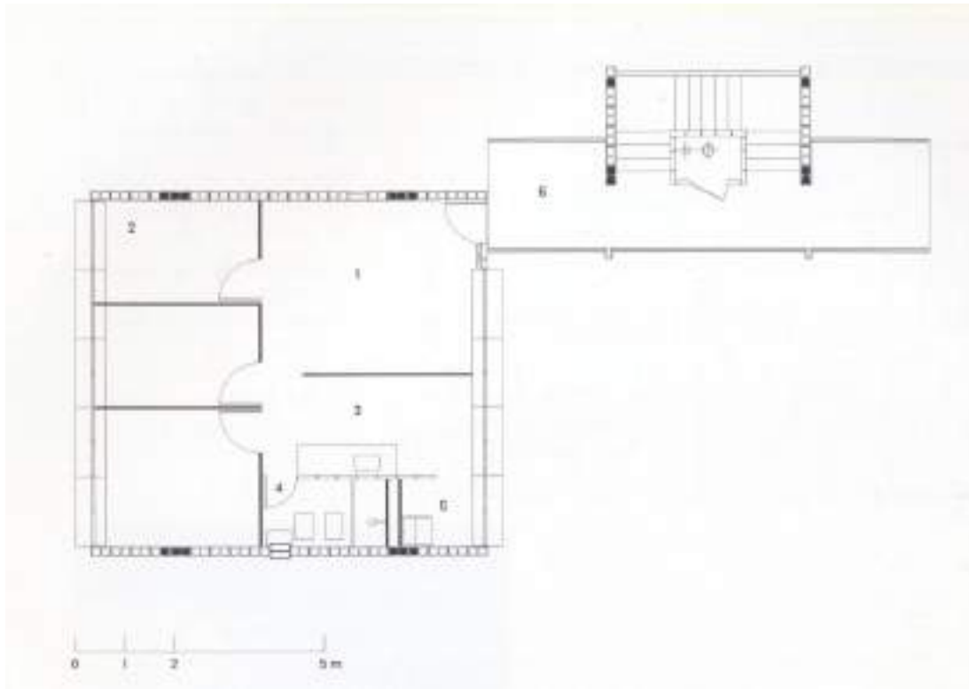
Figura 22. Planta unidad 1ª etapa
