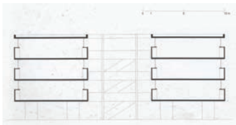
Figura 24. Sección bloque 2ª etapa
